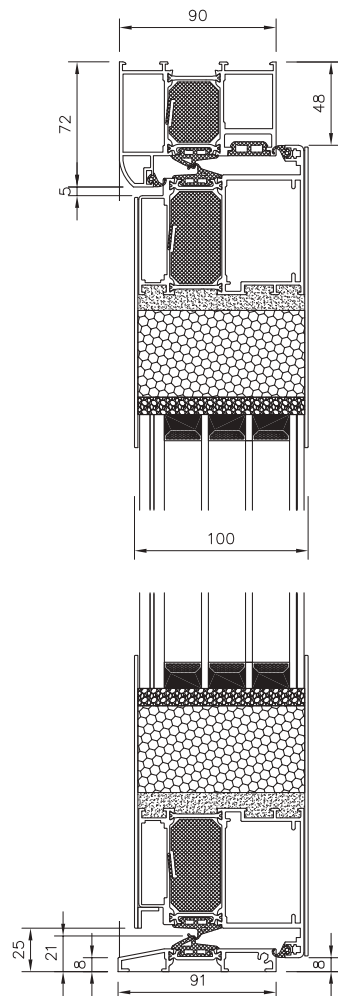
Profilsystem Symphonie, 90 mm
