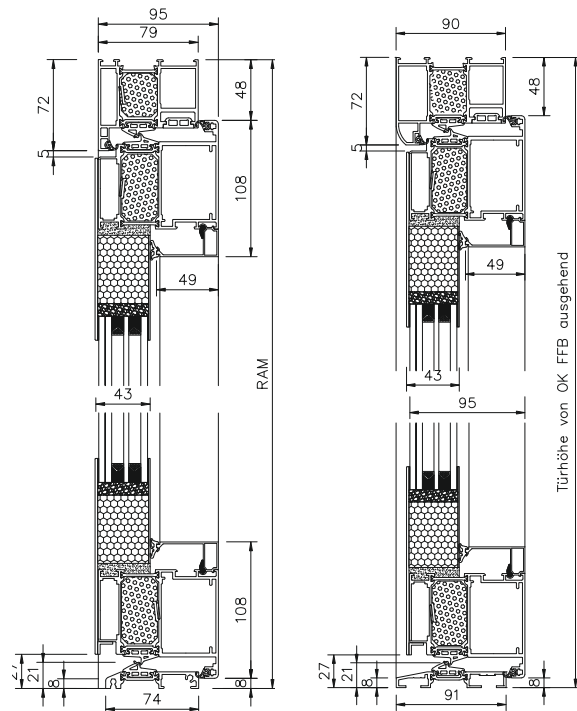
drei dreiteilige Rollenbänder, dreidimensional verstellbar, EV1
