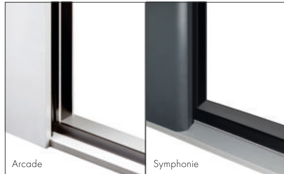
Bodenschwelle thermisch getrennt mit Anschlag- und Mitteldichtung
