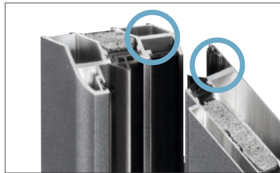
Wandstärke bis 3 mm bietet einen sicheren Halt für Schloss und Bandbolzen
